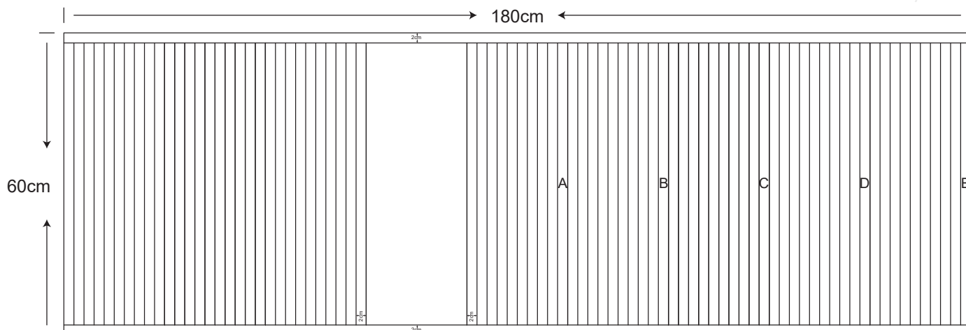
圖 9-3 賽道場地尺寸標示圖
